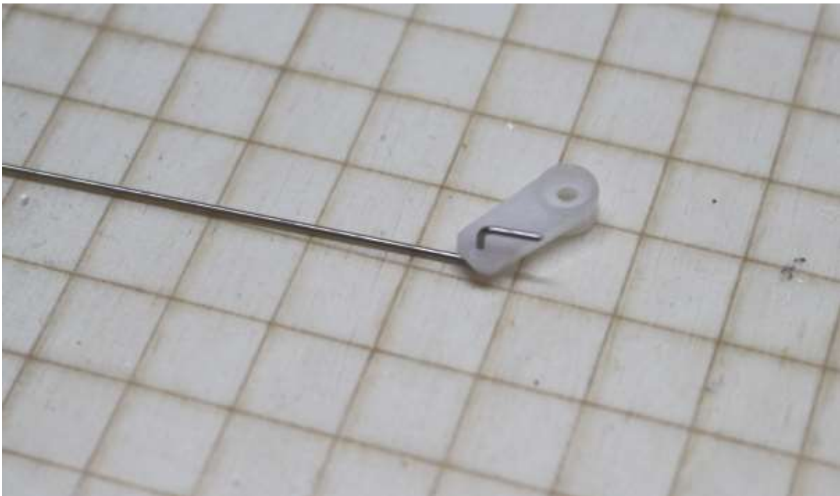
Anlenkungsdraht (Stahldraht \varnothing 0,8 mm) an einem Ende Z-förmig biegen und am Servohebel einhängen
