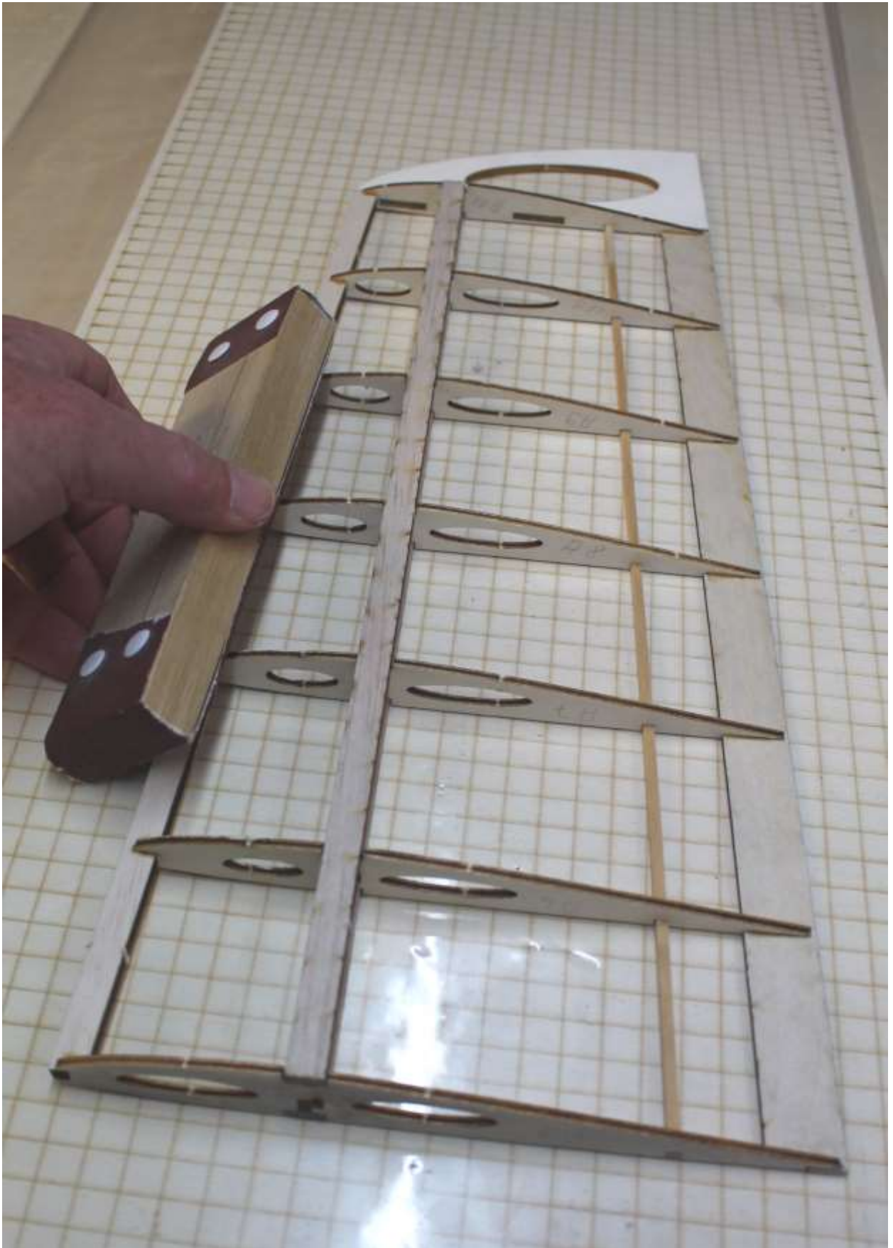
Nasenleiste mit einer langen Schleiflatte verrunden, Tragfläche insgesamt vorsichtig überschleifen
