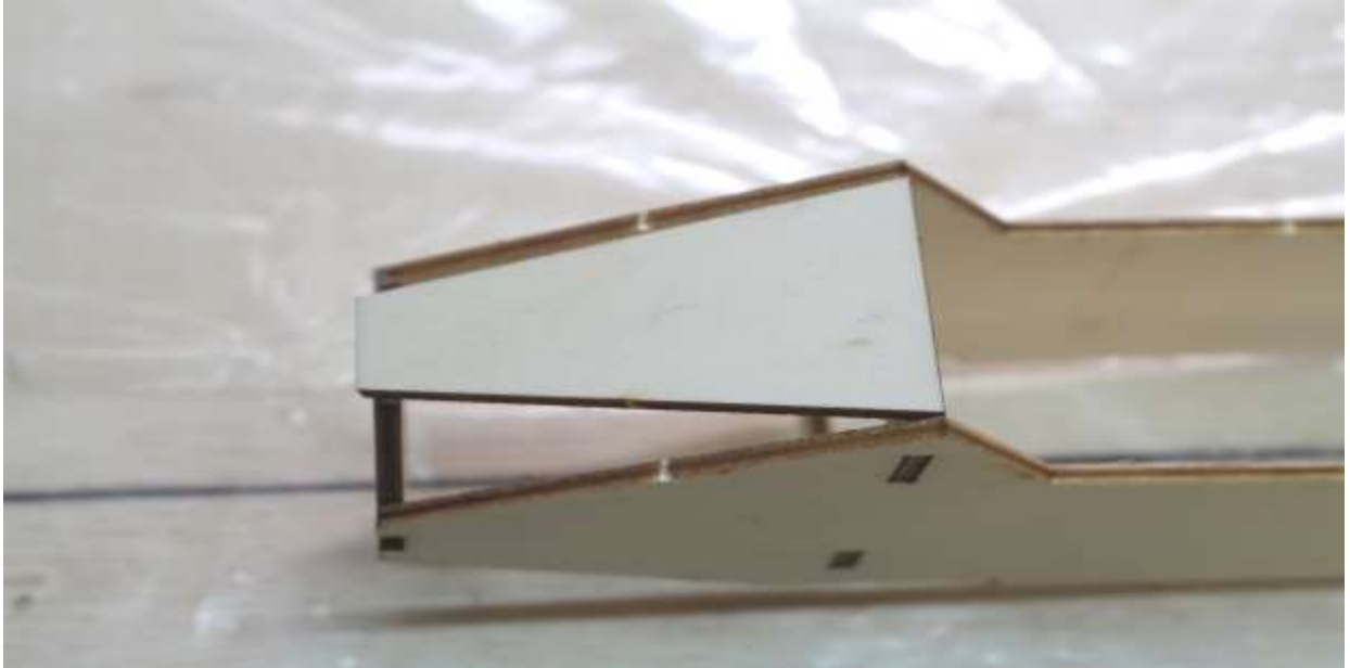
Obere Beplankung der Rumpfspitze (H8) verkleben
