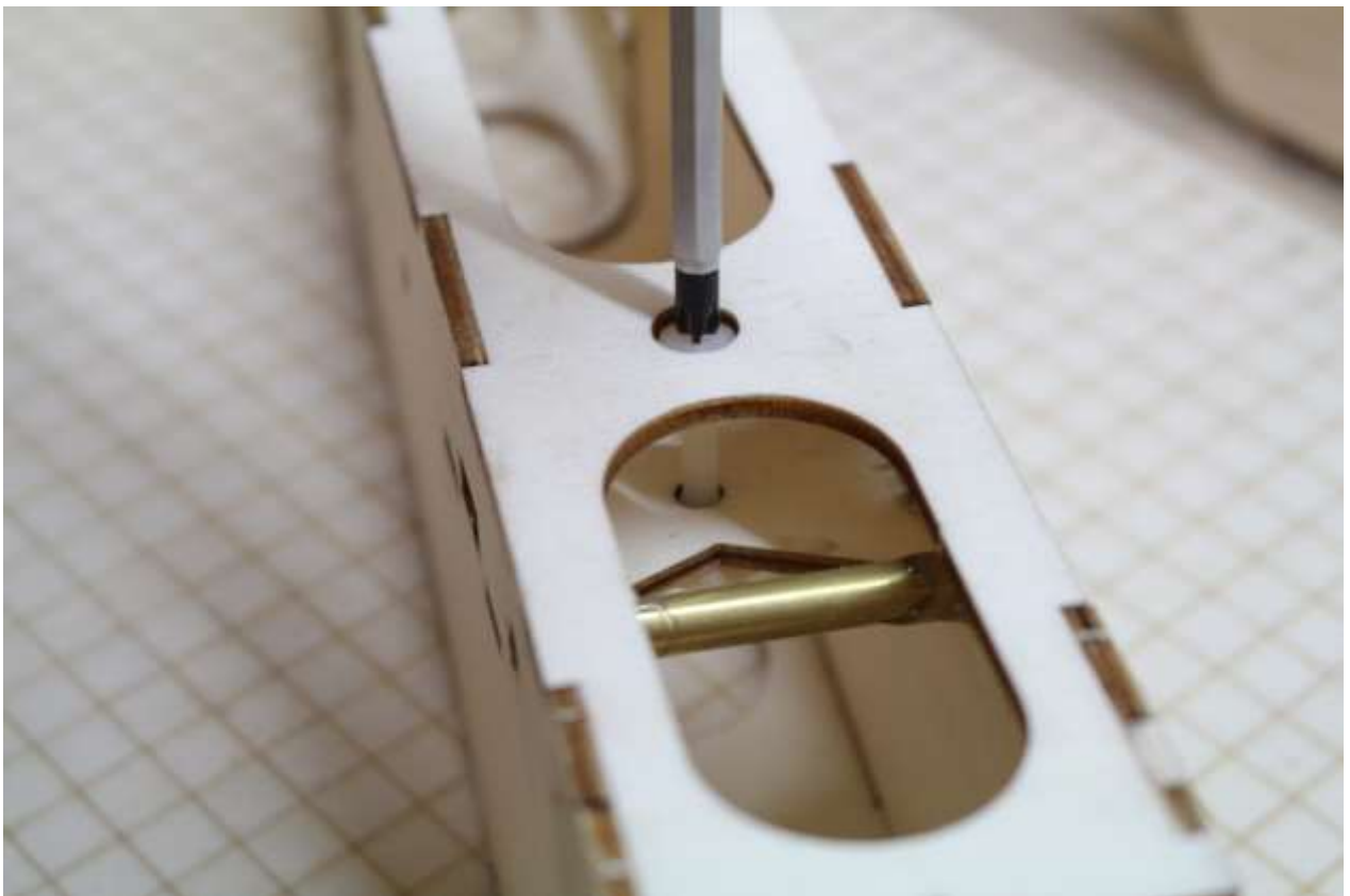
Klemmschraube (Kunststoff M4) für Tragflächensicherung eindrehen
