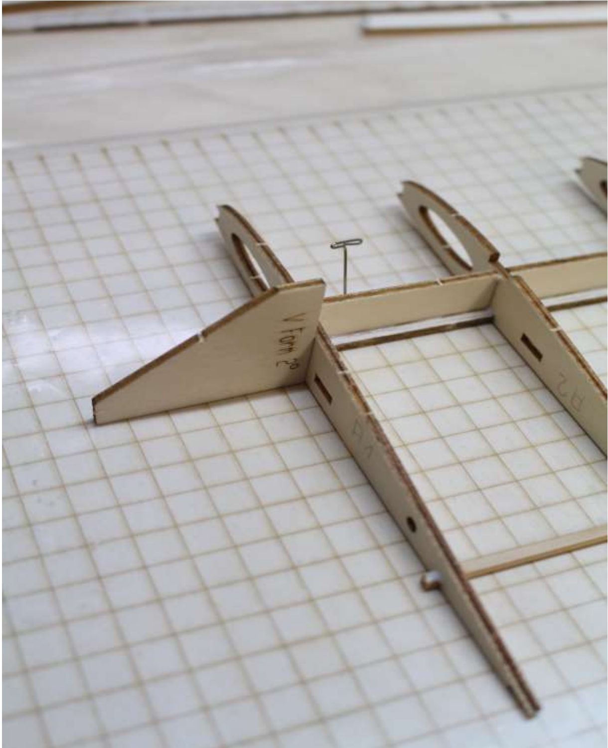
Wurzelrippe mit einer Schräge von 2^\circ verkleben
