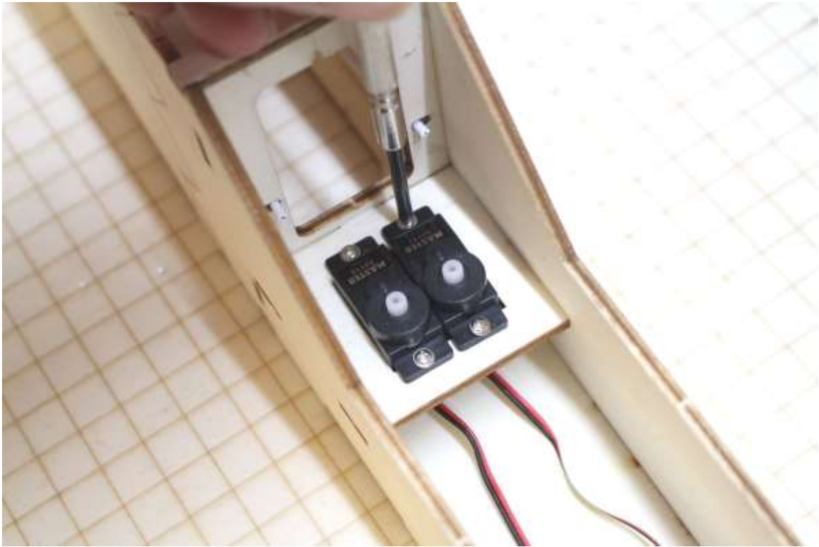
Servos in Servobrett (H6) einsetzen und mit den dem Servo beigelegten Schrauben befestigen
