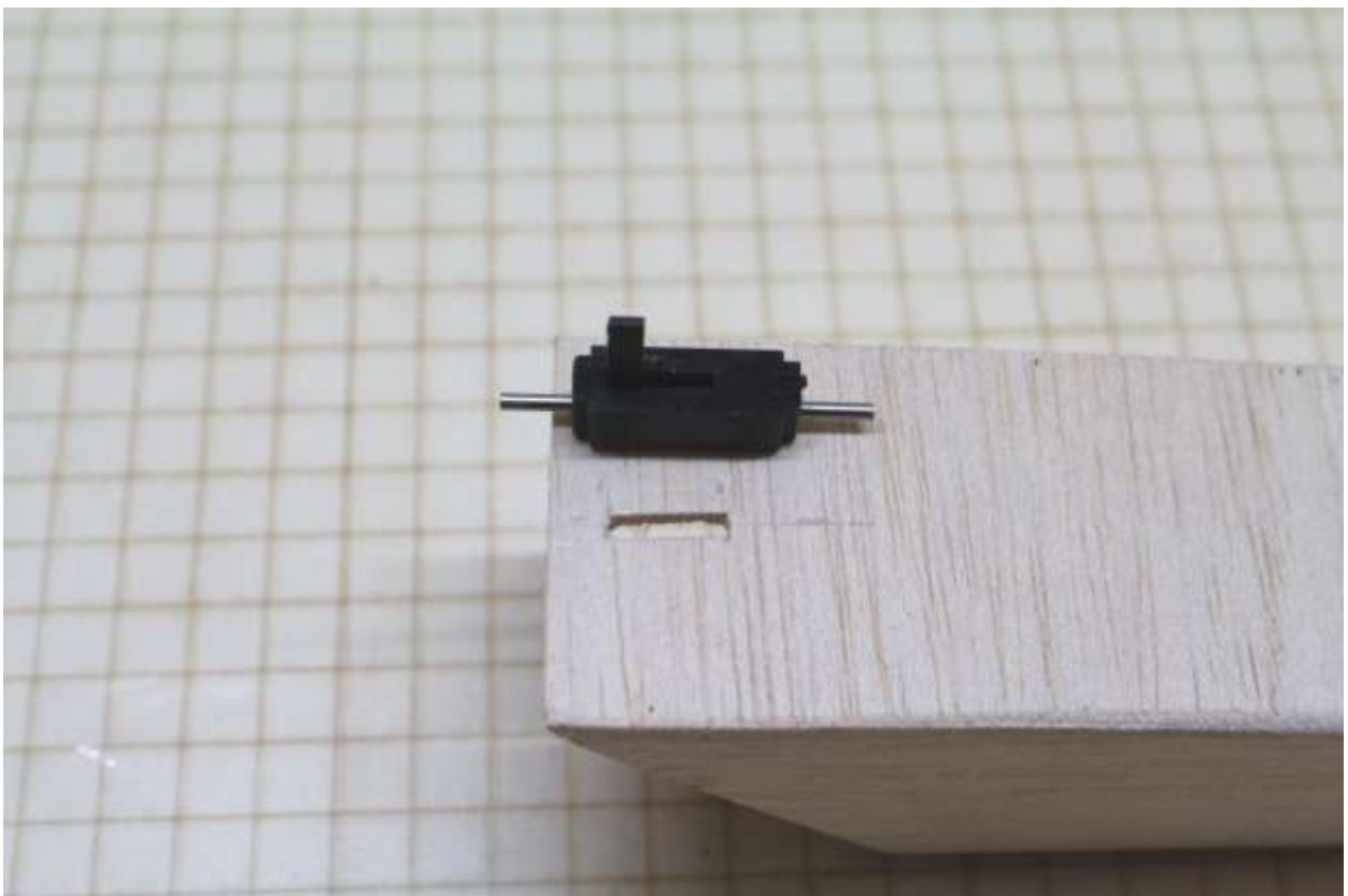
Schlitz für Riegel des Kabinenhaubenschlusses mit einer Breite von 2 mm feilen. ACHTUNG. Form und Ausführung des Kabinenhaubenschlusses kann abweichen.
