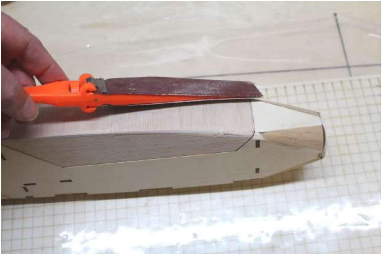
Kabinenhaube auf Rumpf aufsetzen und der Rumpfform verlaufend verschleifen
