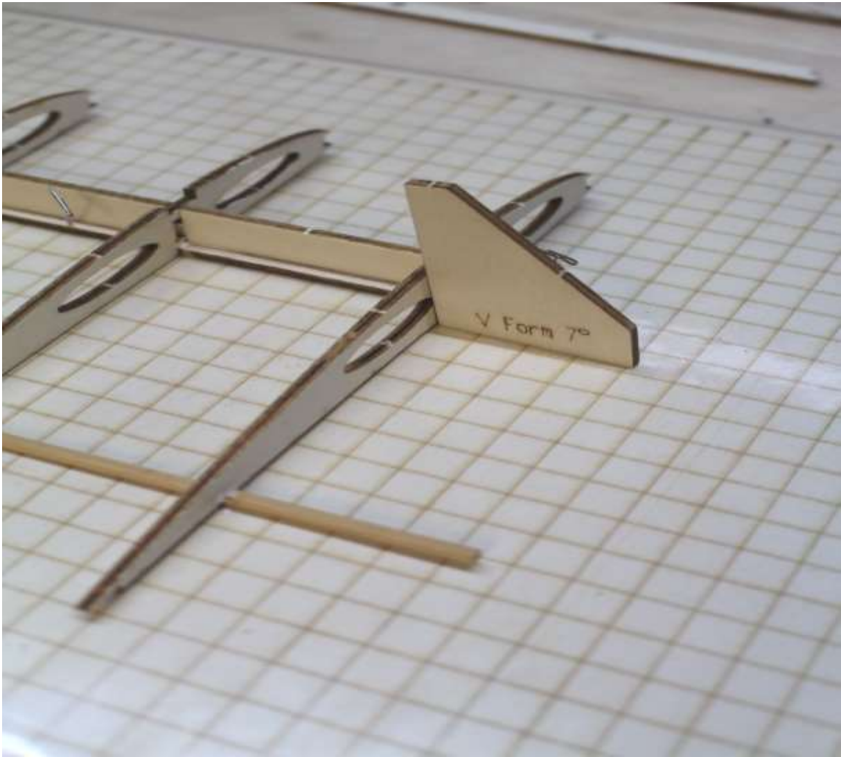
Die Anschlussrippe zum Außenflügel mit 7° verkleben
