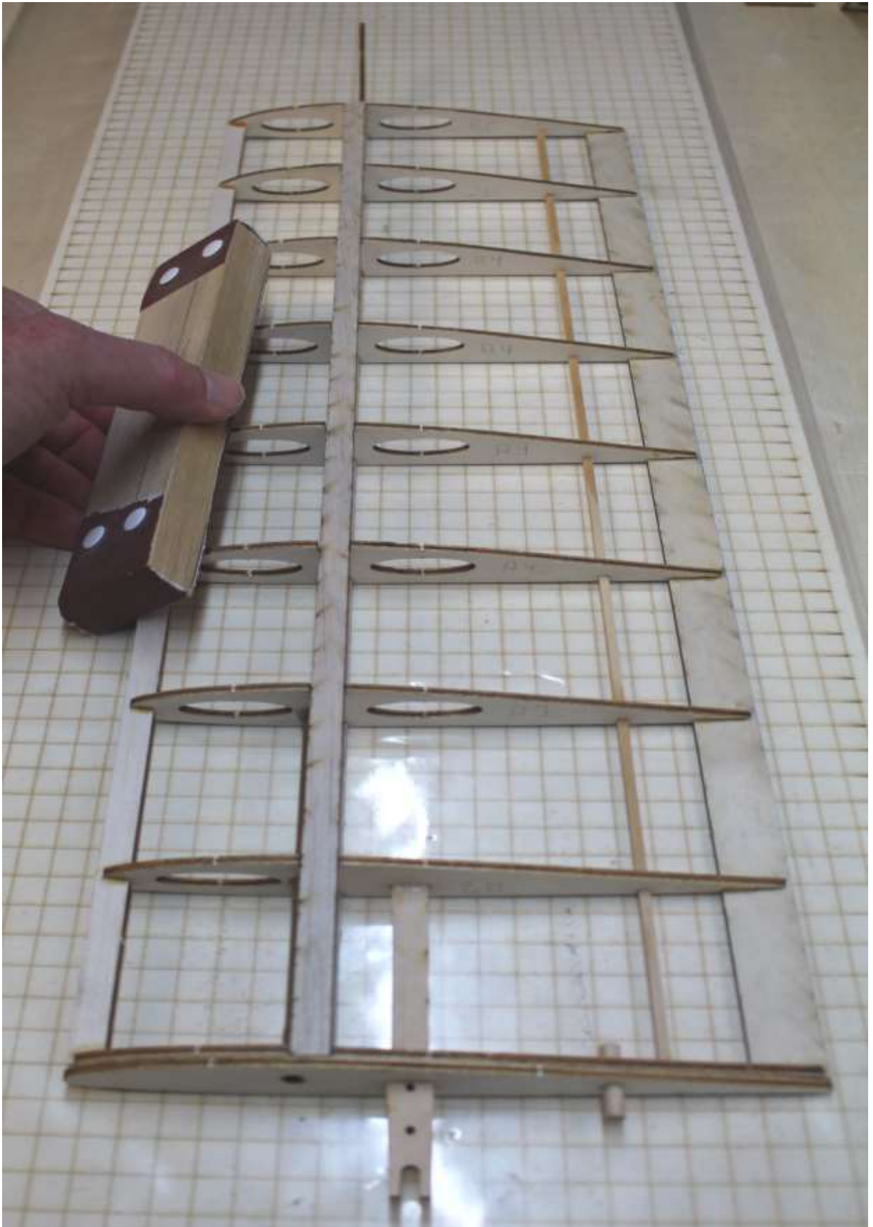
Nasenleiste mit einer langen Schleifplatte verrunden, Tragfläche insgesamt vorsichtig überschleifen
