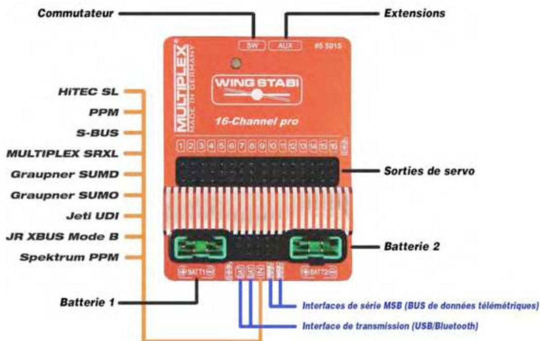
Illustration 4 : WINGSTABI par attribution des branchements
