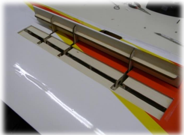
B-) Spoilers up position.
