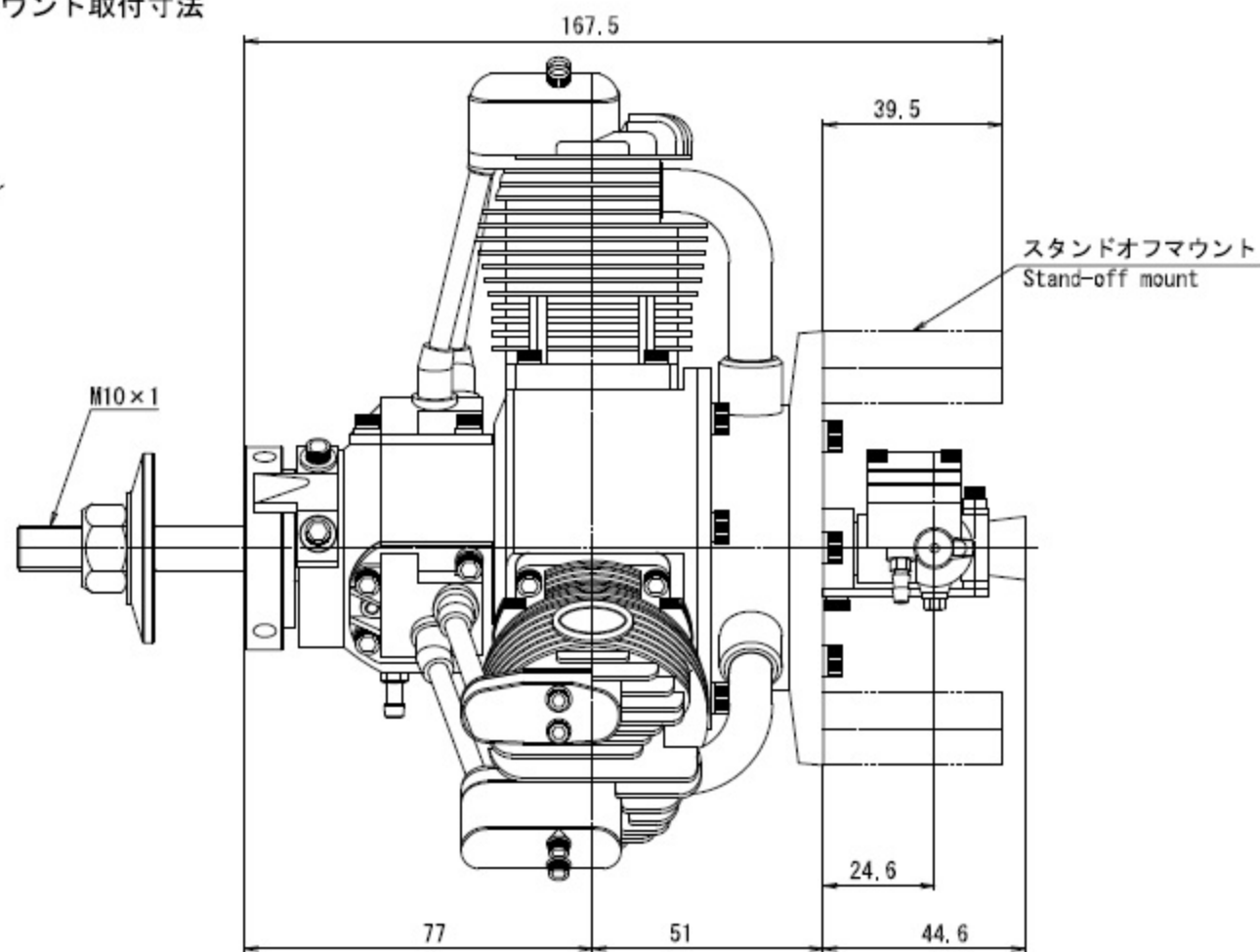
マウント取付寸法
