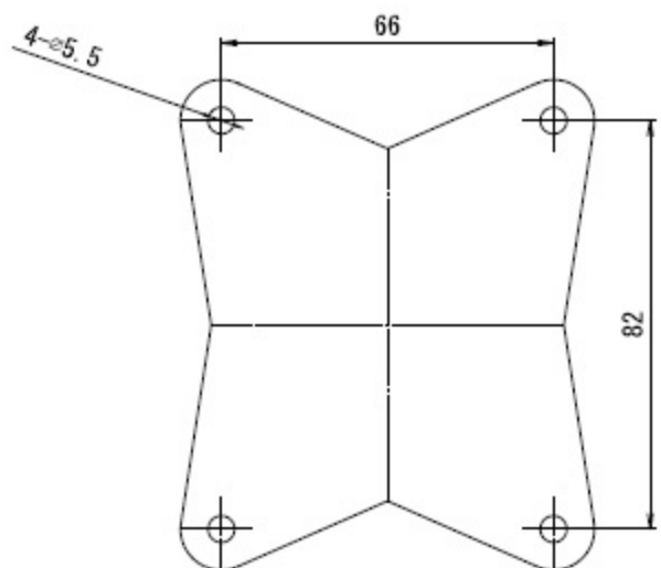
マウント取付寸法
